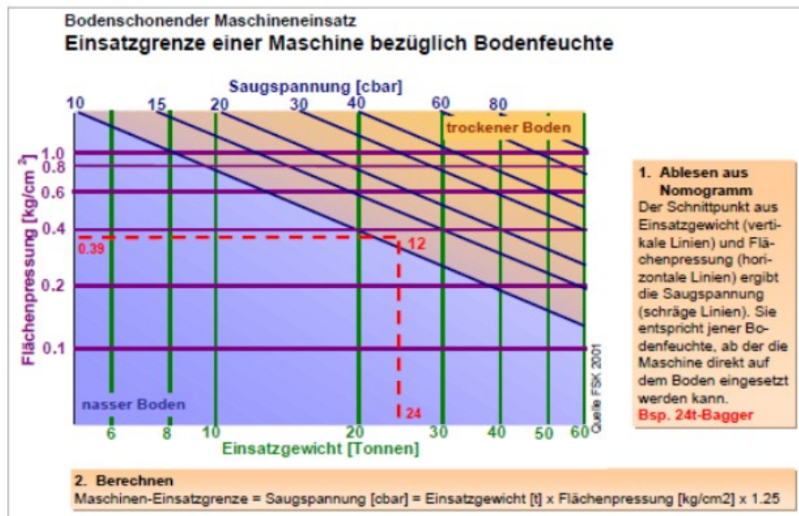
Abb. 11: Einsatzgrenzen von Baumaschinen (AFU 2003)
