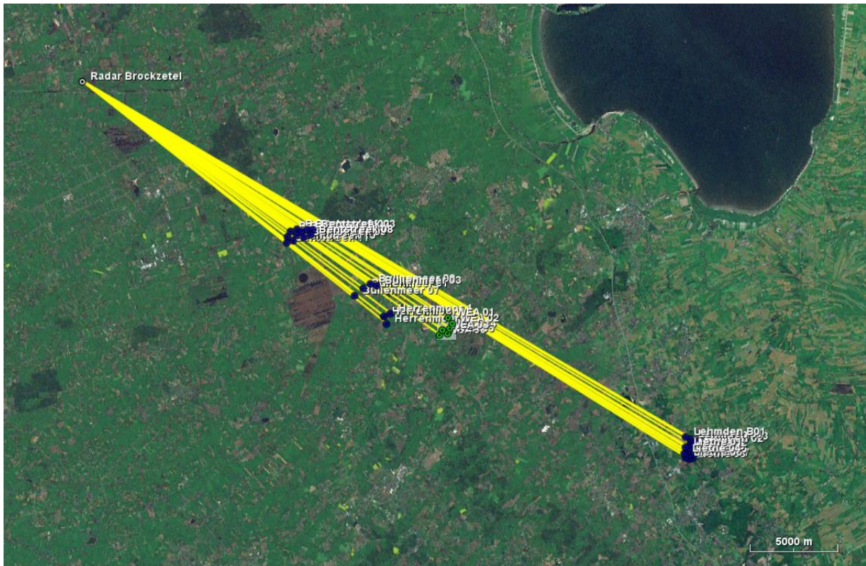
Abbildung 2: Luftaufnahme des Windparks Jühdener Feld mit den geplanten Windenergieanlagen (grün), sowie der berücksichtigten Vorbelastung (blau). Die Einstrahlungsrichtungen bzgl. der Radaranlage Brockzetel sind gelb dargestellt. Um eine bessere Übersicht zu gewährleisten wurden die Bezeichnungen von einzelnen Anlagen teilweise ausgeblendet. Copernicus Sentinel data [2024]
