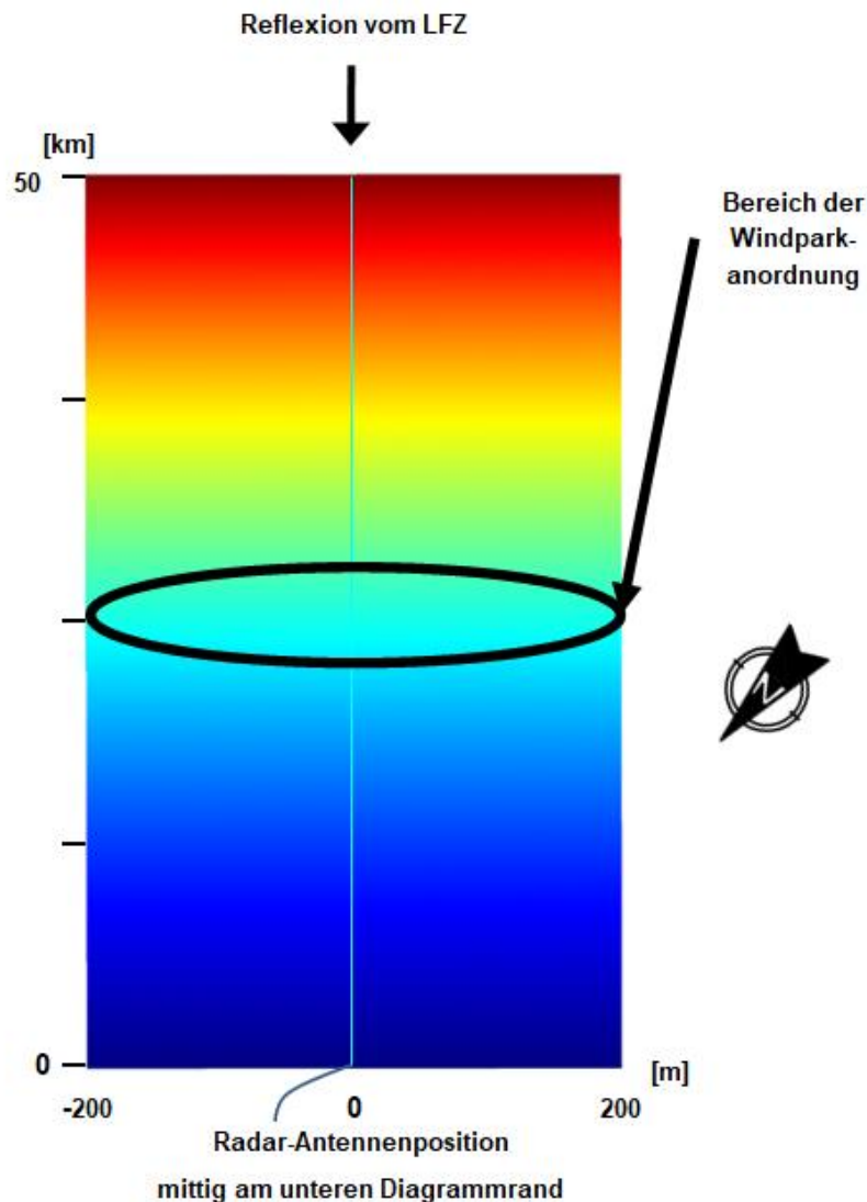
Abbildung 4: Feldgebiet von 50 km x 400 m in der Übersicht (schematische Übersicht für das Radar Brockzetel)
