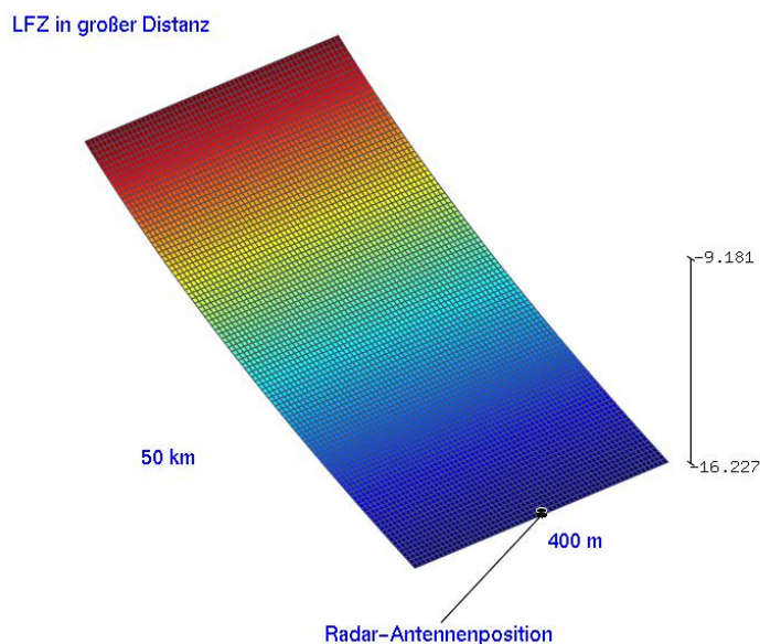
Abbildung 5: Das dargestellte Raumgebiet mit einer Elevation von +0,2^\circ ohne WEA-Einfluss in der Konturdarstellung für die Betriebsfrequenz des Radars Brockzetel
