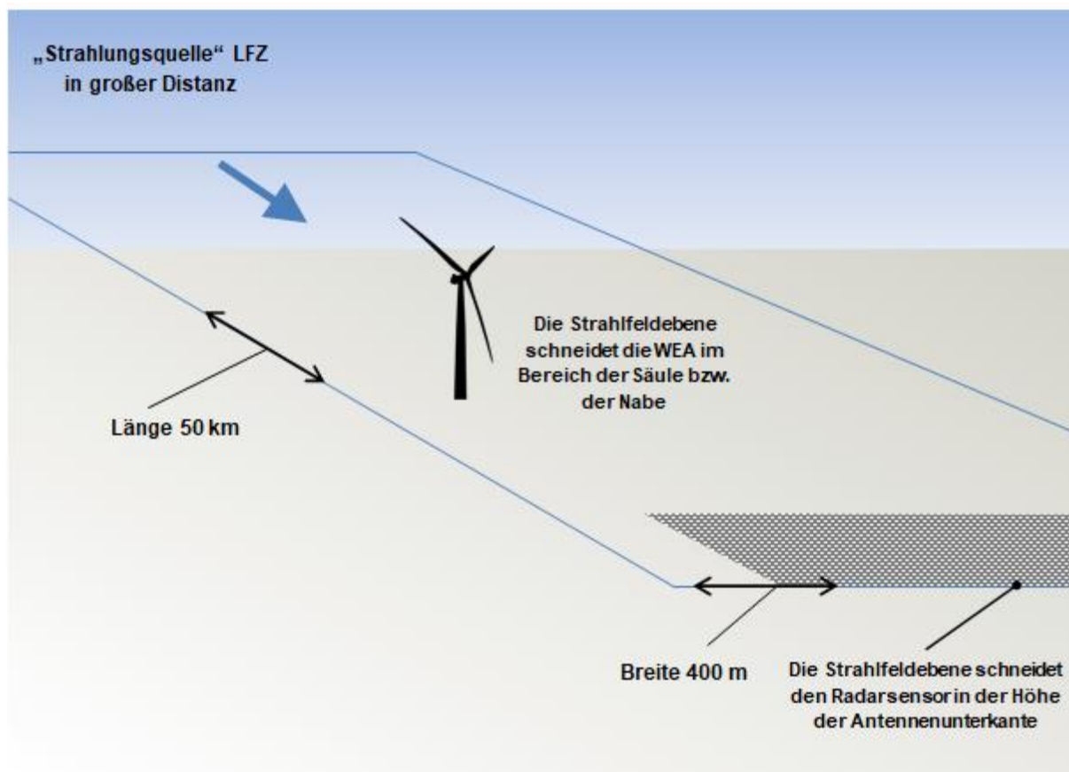
Abbildung 3: Anordnung von Radar und WEA sowie Lage des in dieser Untersuchung dargestellten Luftraums mit einer Ausdehnung von (hier) 50 km x 400 m Breite. Das Lfz wird in einer Distanz von bis zu 130 NM angenommen. – schematische Darstellung –
