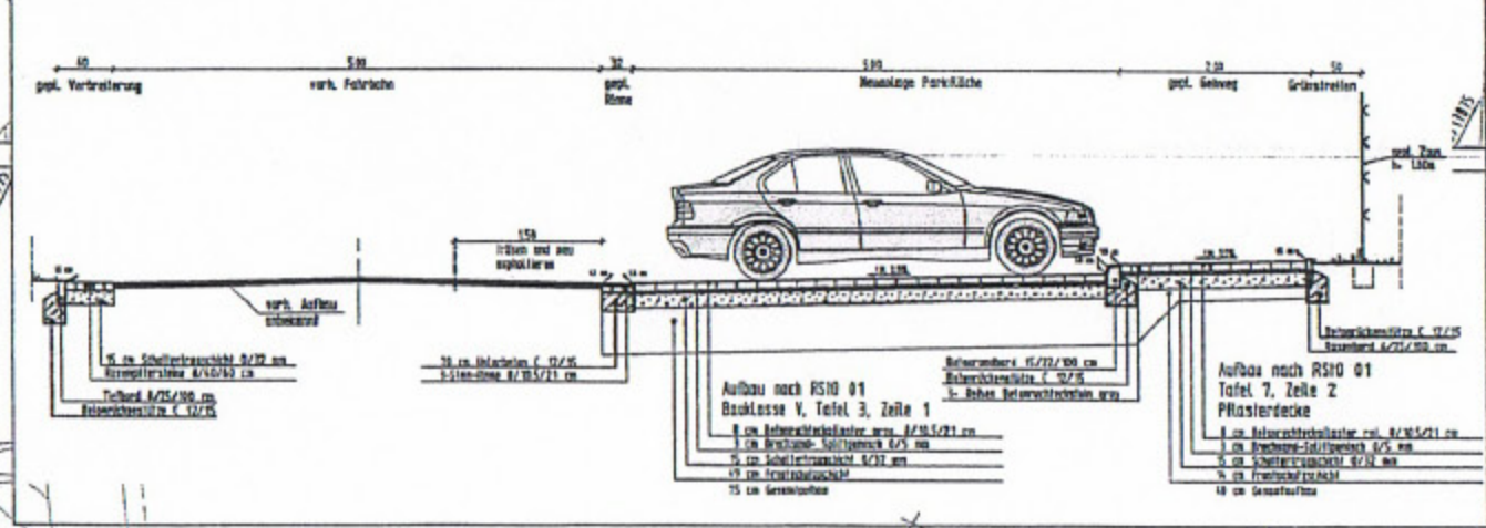
Regelquerschnitt Parkstreifen H. 1.50
